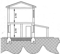
SEZIONE VERTICALE
