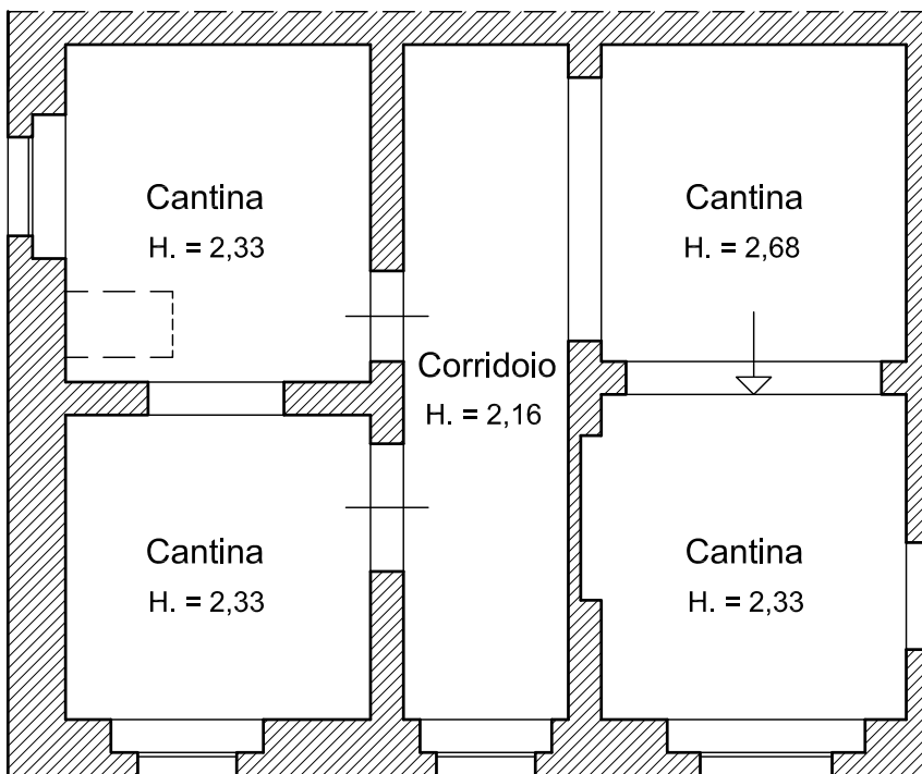
Primo piano sottostrada
